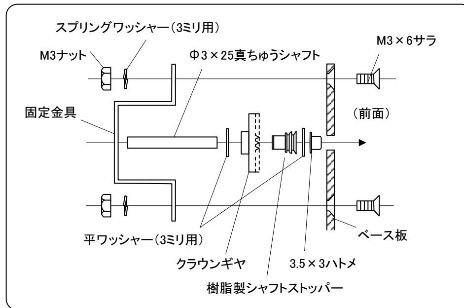
■出力軸の組み立て図
